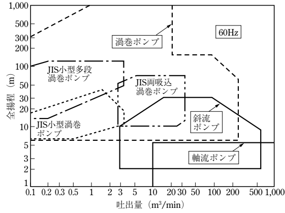
ポンプ形式選定図 (60Hz用)
