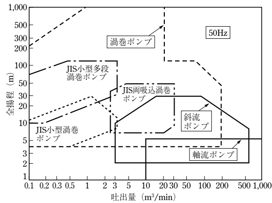
ポンプ形式選定図 (50Hz用)
